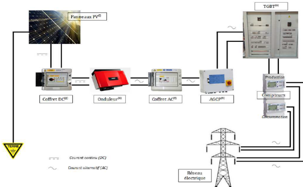
Schéma de principe d'un système photovoltaïque
